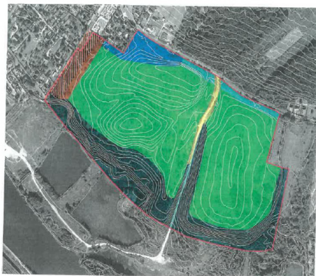
Carte des préconisations paysagères pour le projet de centrale photovoltaïque
